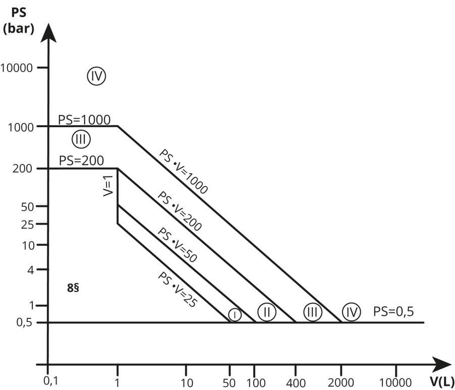
Diagram 1: Tryckkärl som avses i 6 § a) i. första strecksatsen
