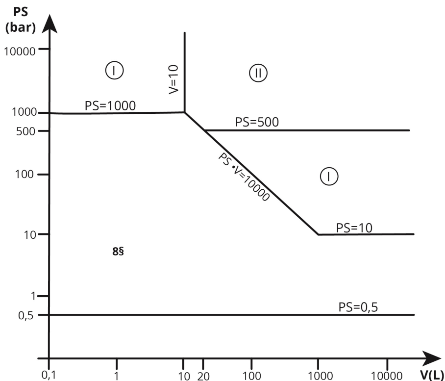
Diagram 4: Tryckkärl som avses i 6 § a) ii. andra strecksatsen
