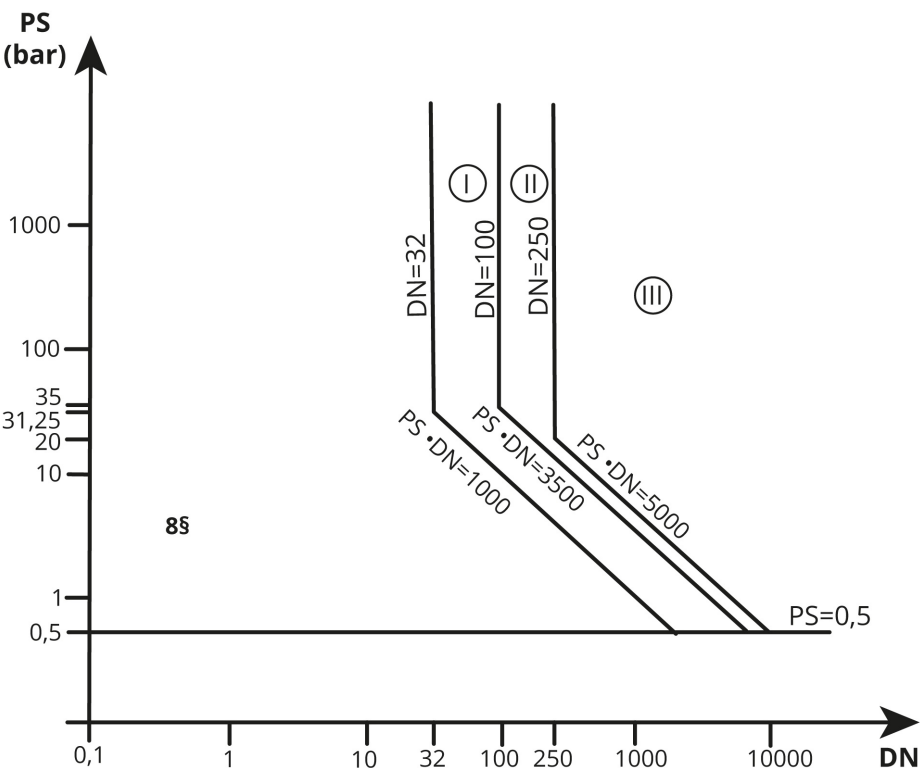
Diagram 7: Rörledningar som avses i 6 § c) i. andra strecksatsen
