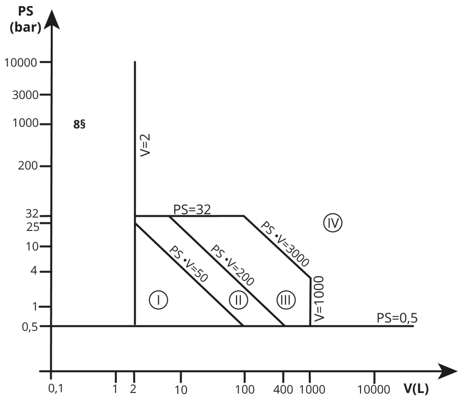
Diagram 5: Tryckbärande anordningar som avses i 6 § b)
