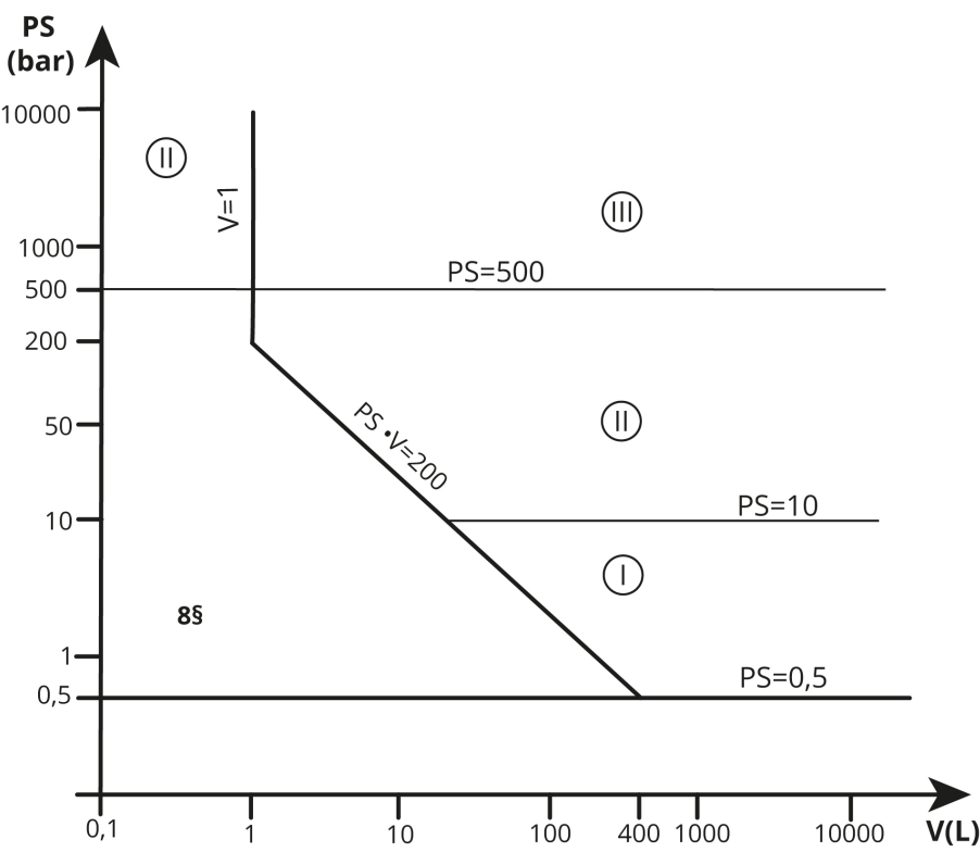
Diagram 3: Tryckkärl som avses i 6 § a) ii. första strecksatsen
