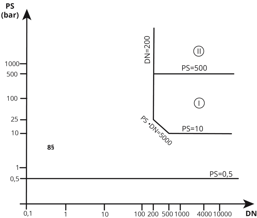
Diagram 9: Rörledningar som avses i 6 § c) ii. andra strecksatsen
