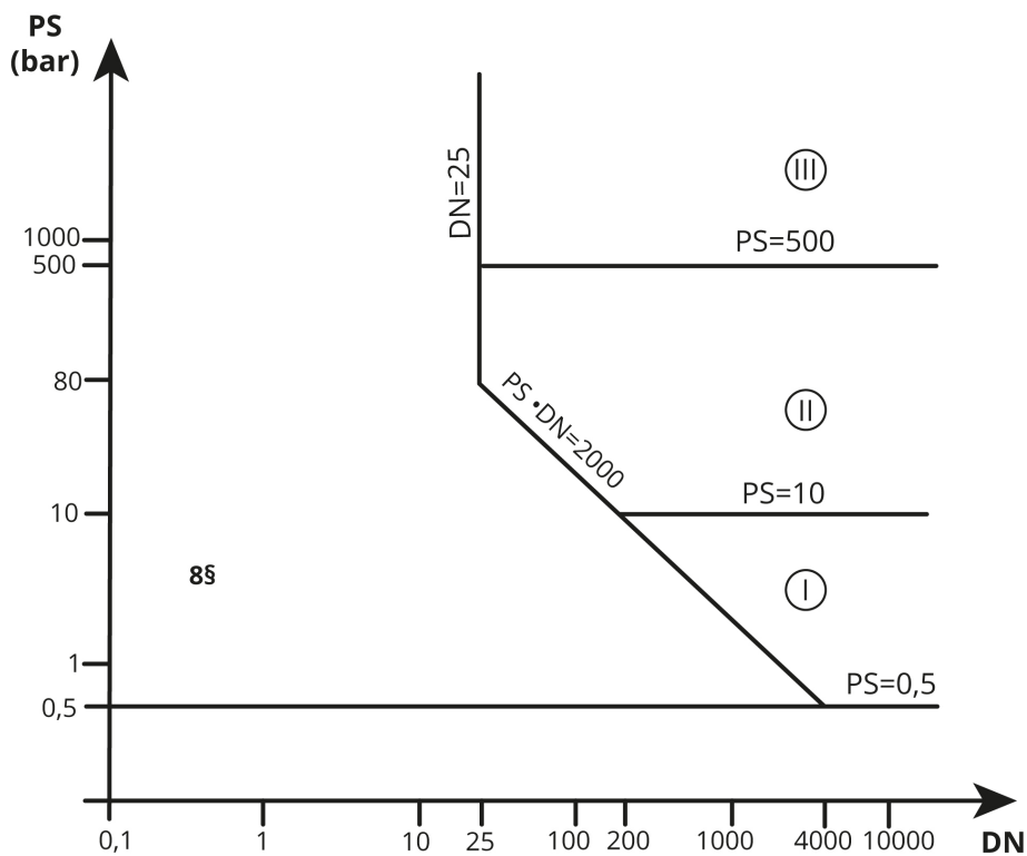
Diagram 8: Rörledningar som avses i 6 § c) ii. första strecksatsen
