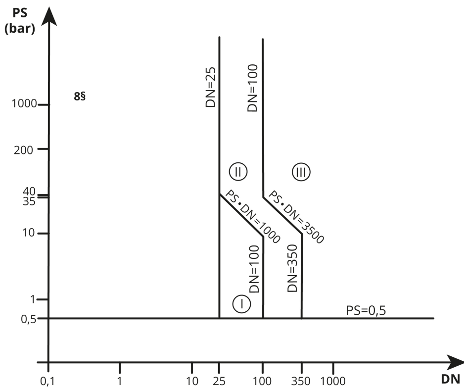
Diagram 6: Rörledningar som avses i 6 § c) i. första strecksatsen
