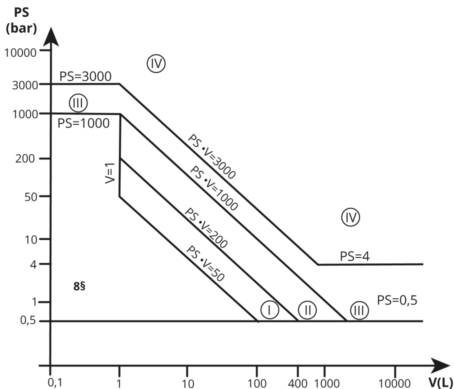
Diagram 2: Tryckkärl som avses i 6 § a) i. andra strecksatsen
